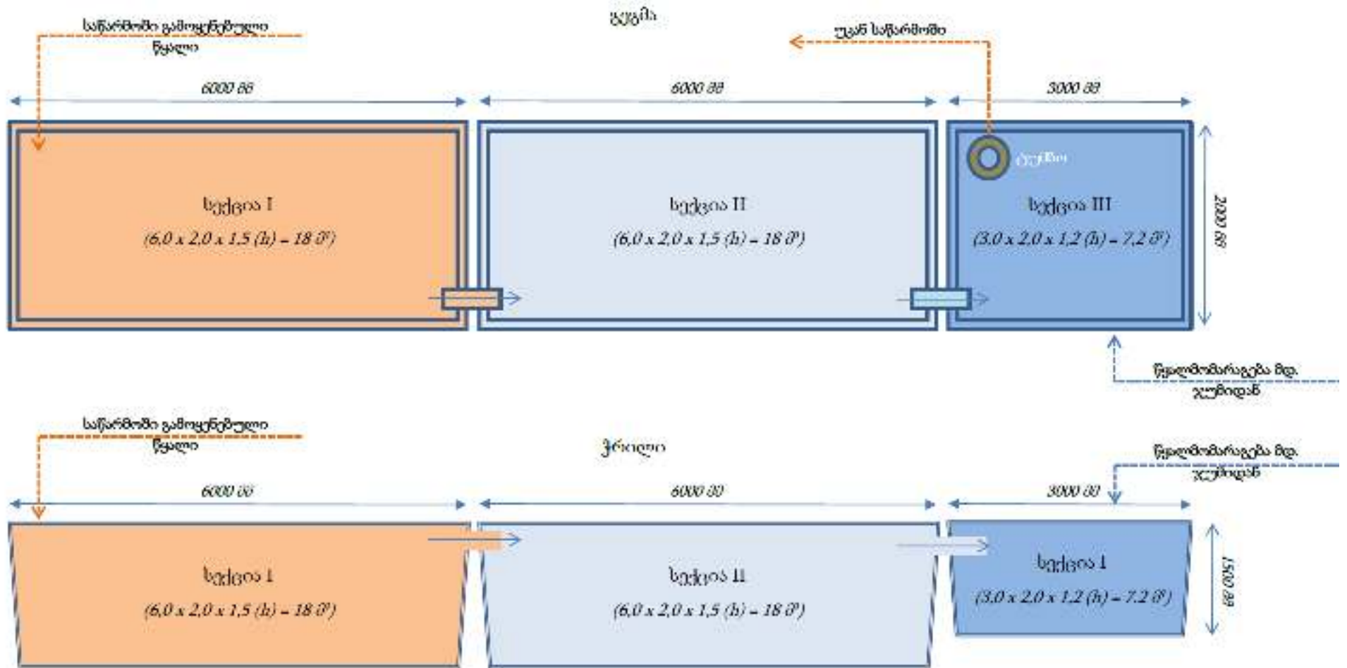
ნახაზი 2.2.3.1. საწარმოში დაგეგმილი სალექარის გეგმა და ქრილი
